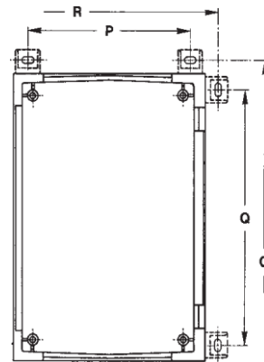
Монтаж на стіну зі скобами з поліаміду
