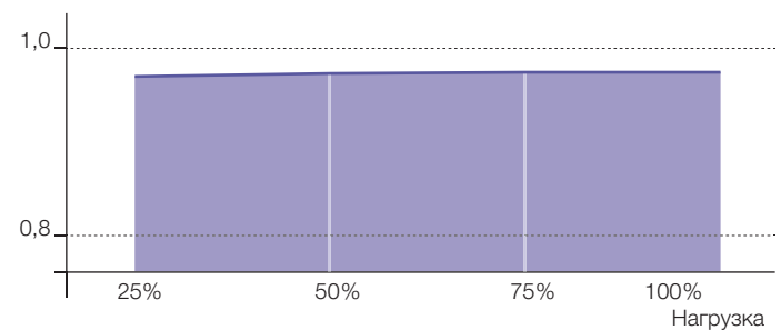
Входной коэффициент мощности в зависимости от нагрузки
